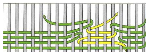
Закрепление утков на общей нити основы
